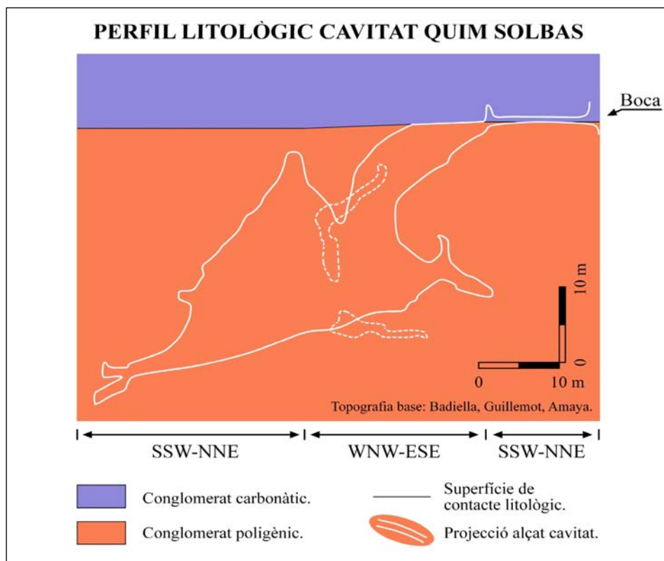
Figura 1: Perfil litològic de la cavitat Quim Solbas.
