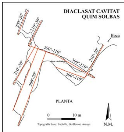
Figura 3: Esquema de la xarxa de diàclasis de la cavitat Quim Solbas.
